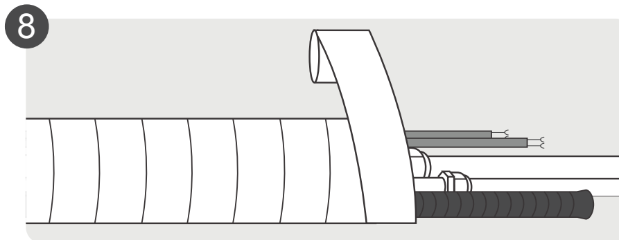
Подготовьте трубопроводы к эксплуатации
