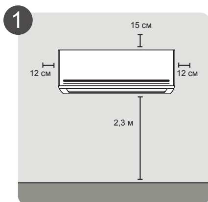
Выберите место монтажа внутреннего блока
