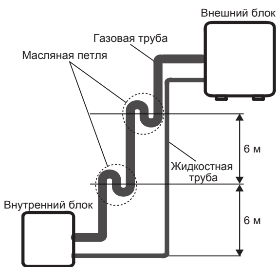
2. Внешний блок установлен выше внутреннего блока
