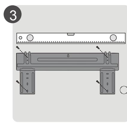
Закрепите монтажную пластину внутреннего блока
