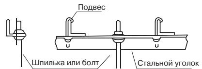
(Подвес трубопровода или блока)
