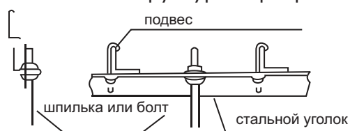
скользящая установка
