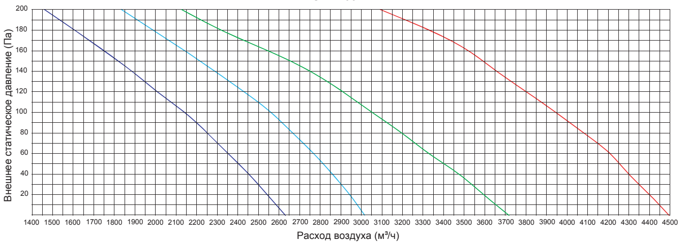
LSF-2200DD22H
