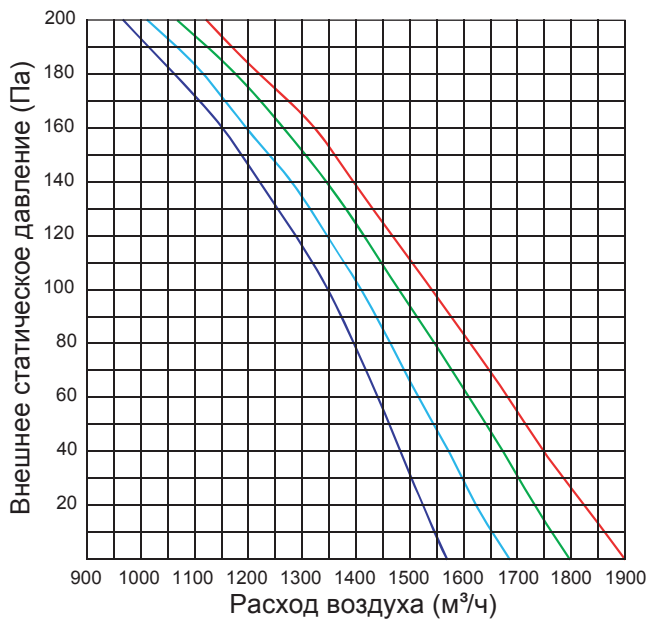
LSF-1400DD22H
