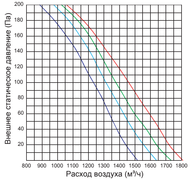
LSF-1000DD22H LSF-1200DD22H
