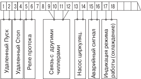
Клеммная колодка поз. X чиллеров LUC-SSAA380/500/600/720CXH
