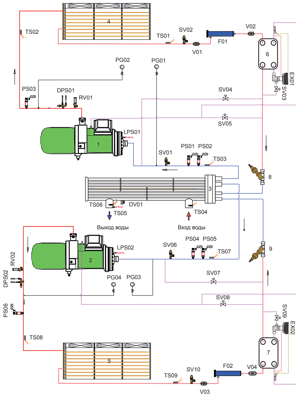
Рис. 3.4. Принципиальная гидравлическая схема контура хладагента винтовых чиллеров LUC-SSDA1200/1420CXH с воздушным охлаждением конденсатора
