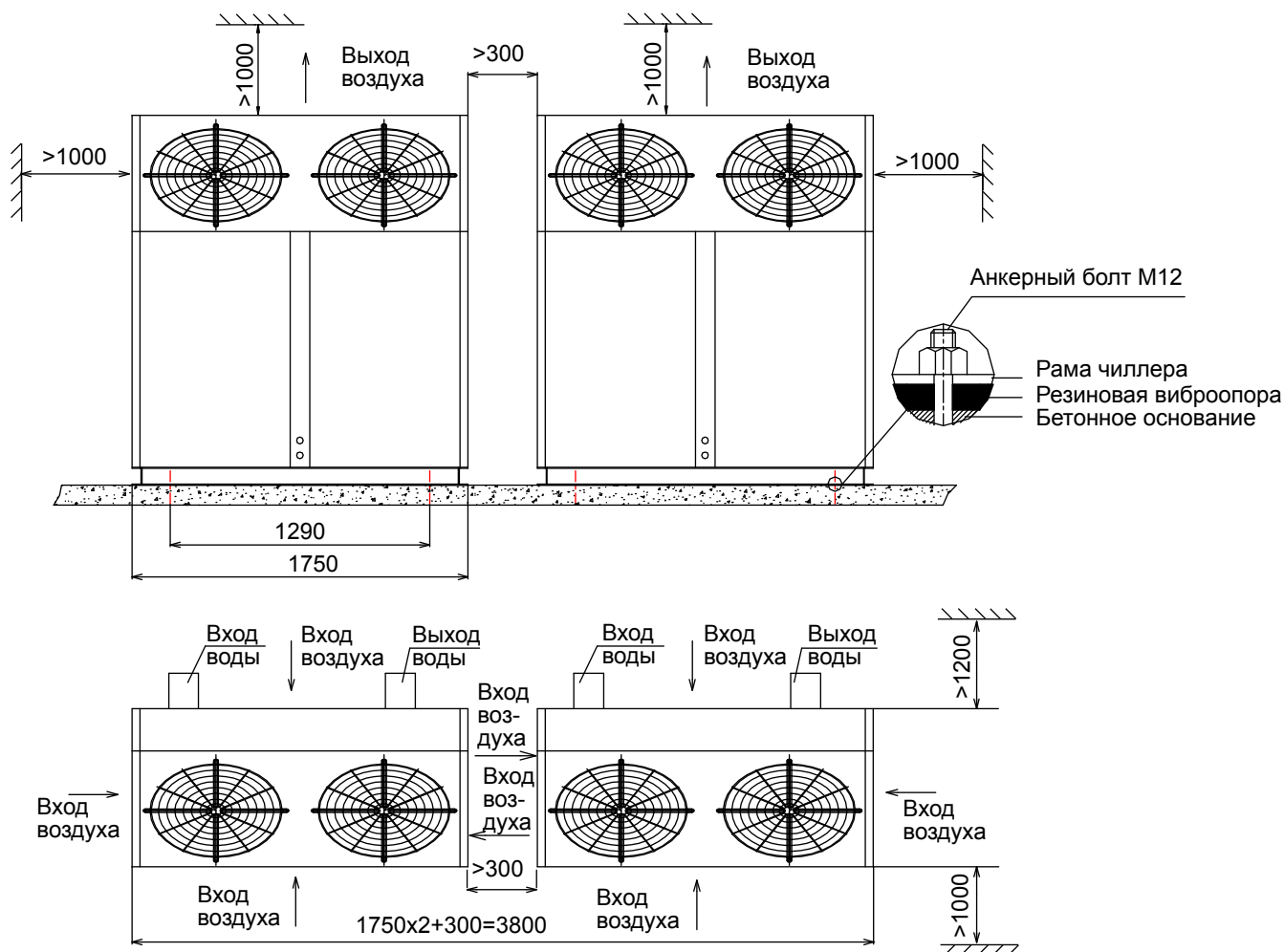
Рис. 2. Установка чиллера на фундамент
