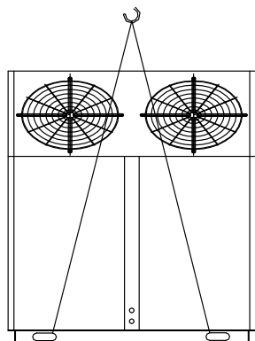
Рис. 1. Строповка чиллера
