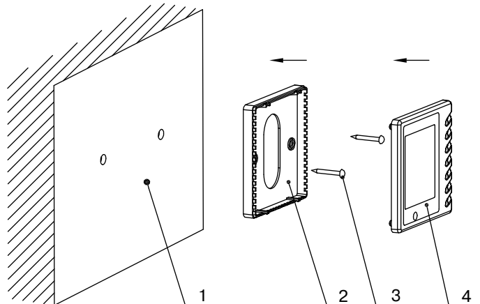
1 — стена; 2 — задняя крышка; 3 — винт M4×10; 4 — передняя панель
