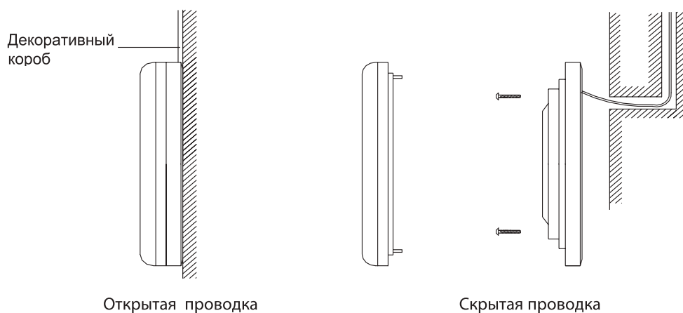
Рис. 14.1 — Установка пульта управления
