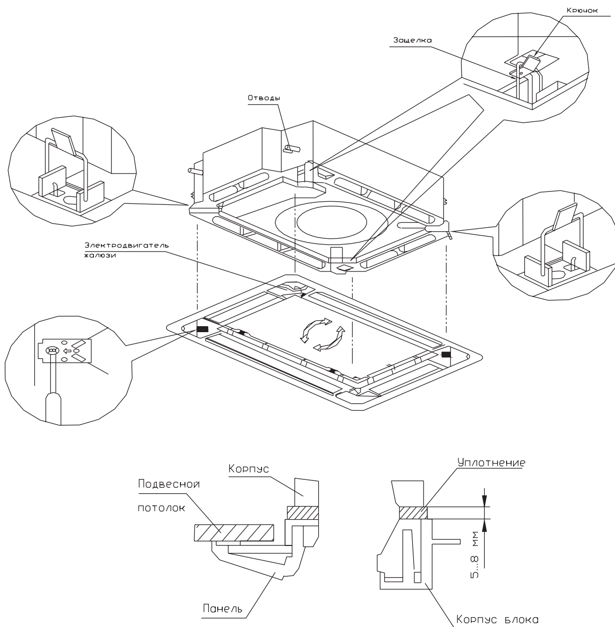
Рис. 10.20 — Установка панели
