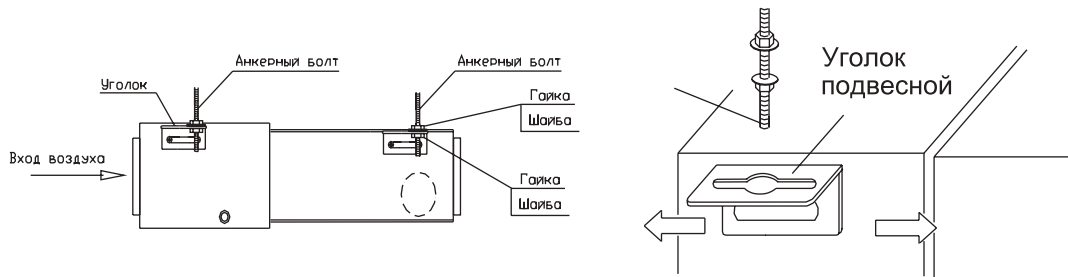
Рис. 10.26 — Установка блока
