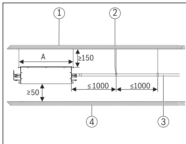
Рис. 1 Минимальные расстояния от группового MS-Vox в мм
