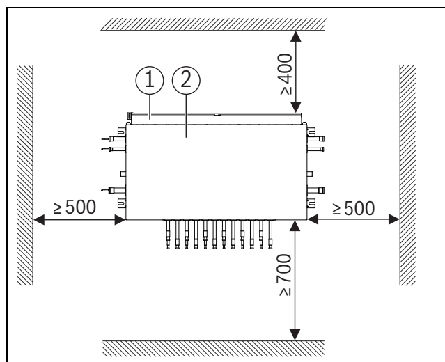
Рис. 2 Минимальные расстояния от группового MS-Vox в мм, вид сверху
