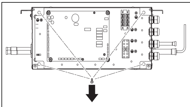
Рис. 8 Перестановка электрического блока с одной стороны на другую (шаг 3)
