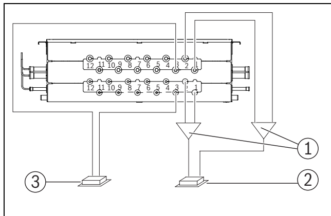
Рис. 23 Подключение MS-Vox к блокам
