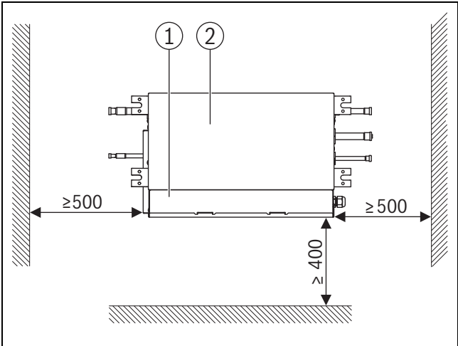
Рис. 4 Минимальные расстояния от группового MS-Vox в мм, вид сверху
