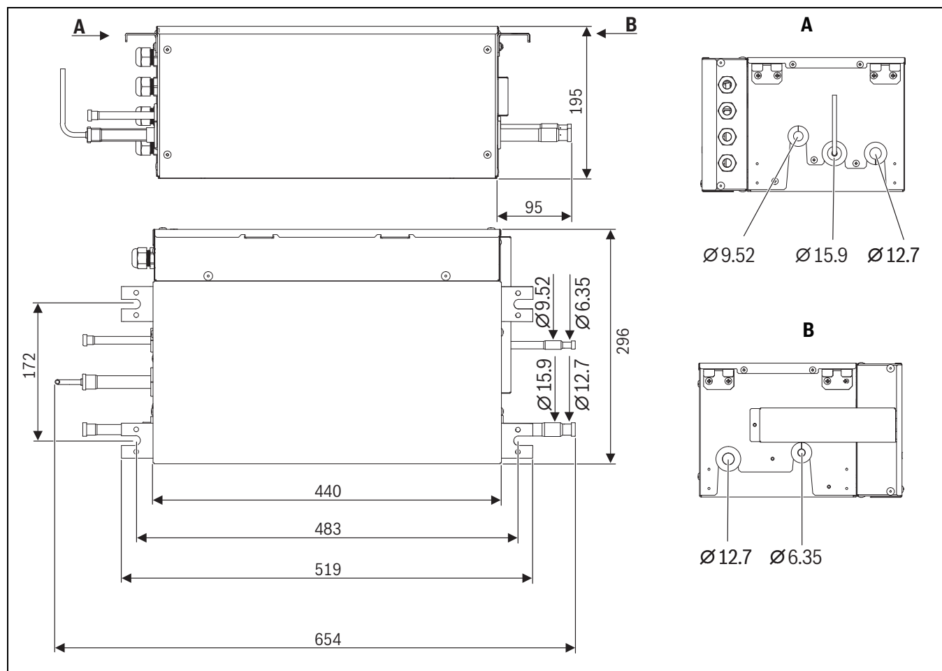
Рис. 21 Размеры одиночного MS-Box в мм
