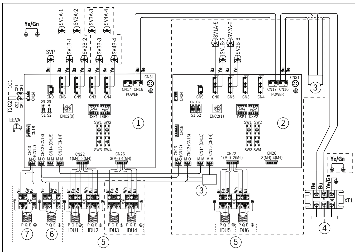
Рис. 40 Схема электрических соединений группового MS-Box
