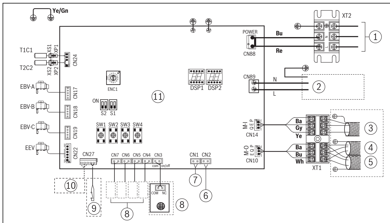
Рис. 39 Схема электрических соединений отдельного MS-Box
