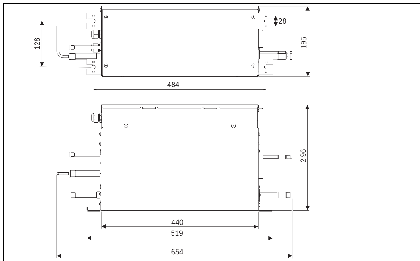
Рис. 22 Размеры одиночного MS01N1-D (настенный монтаж) в мм
