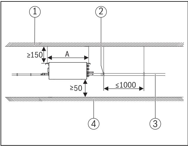
Рис. 3 Минимальные расстояния от одиночного MS-Vox в мм
