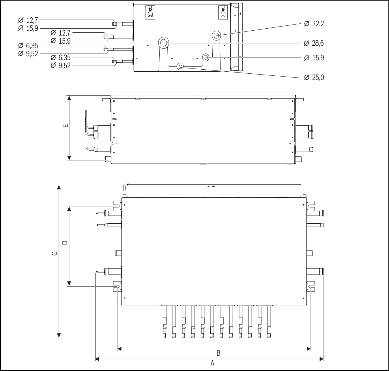
Рис. 20 Размеры группового MS-Box в мм
