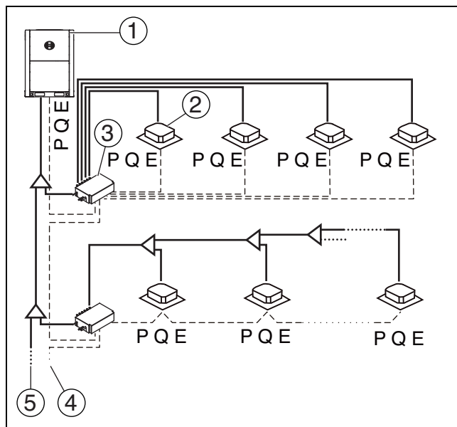
Рис. 42 Электропроводка и трубопроводы блока MS-Box
