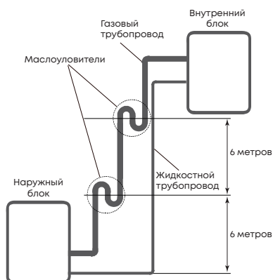
Наружный блок расположен ниже
