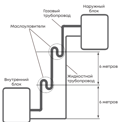
Наружный блок расположен выше
