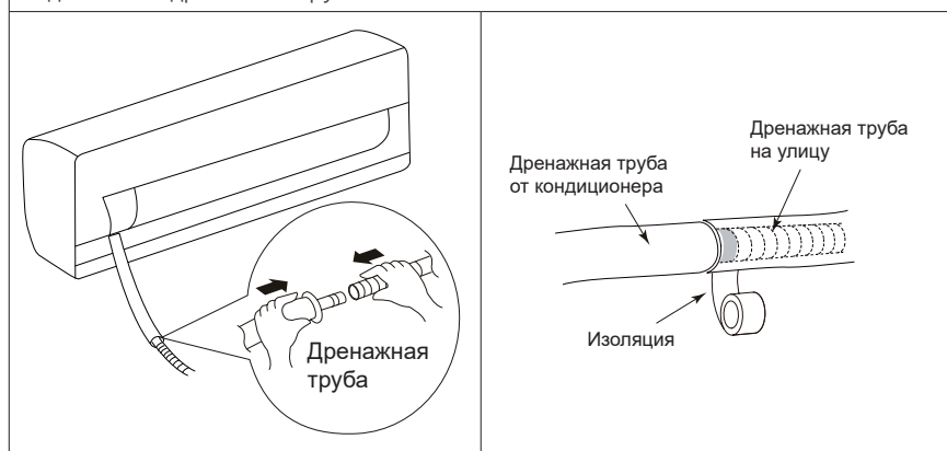
Подключение дренажной трубы
