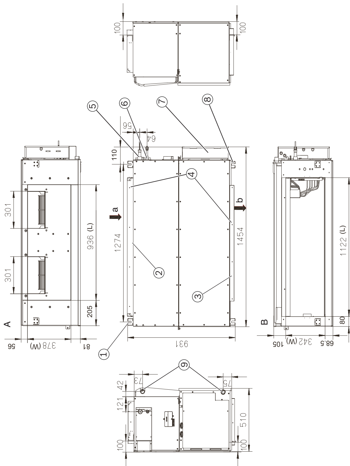
Рис. 11 Размеры прототипов: 20,0 - 25,0 - 28,0
