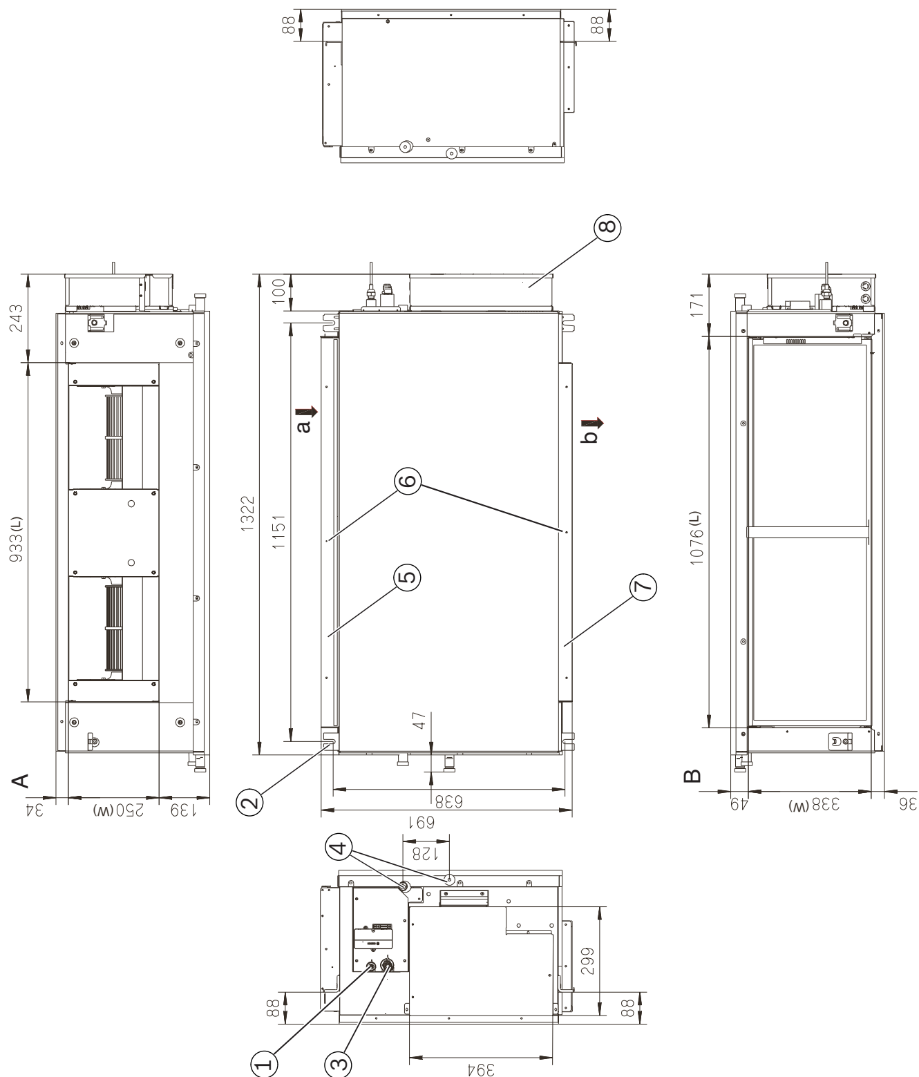
Рис. 10 Размеры прототипов: 14,0 - 16,0
