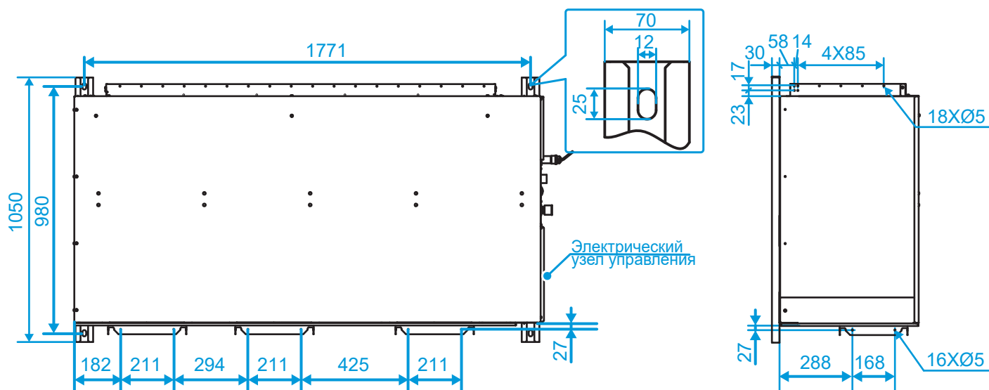
Размеры проушины и резьбового отверстия фланца подачи/забора воздуха:
