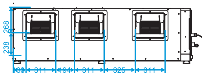
Размеры воздуховыпускного отверстия:
