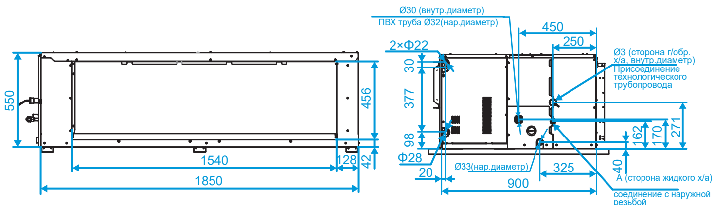
Размеры воздуховыпускного отверстия:
