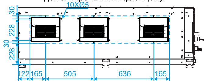
Размеры монтажного отверстия воздуховода (с демонтированным фланцем):
