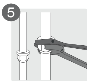
Подключите трубопроводы
