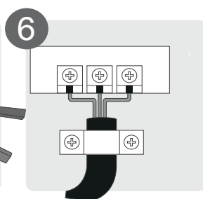
Подключите провода
